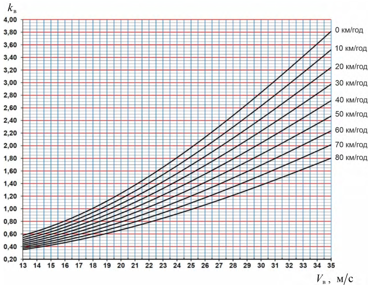
Рис. В.7. Номограма для визначення коефіцієнту k_B за швидкістю вітру від 13 до 35 м/с та густиною повітря 1,5 кг/м 3
