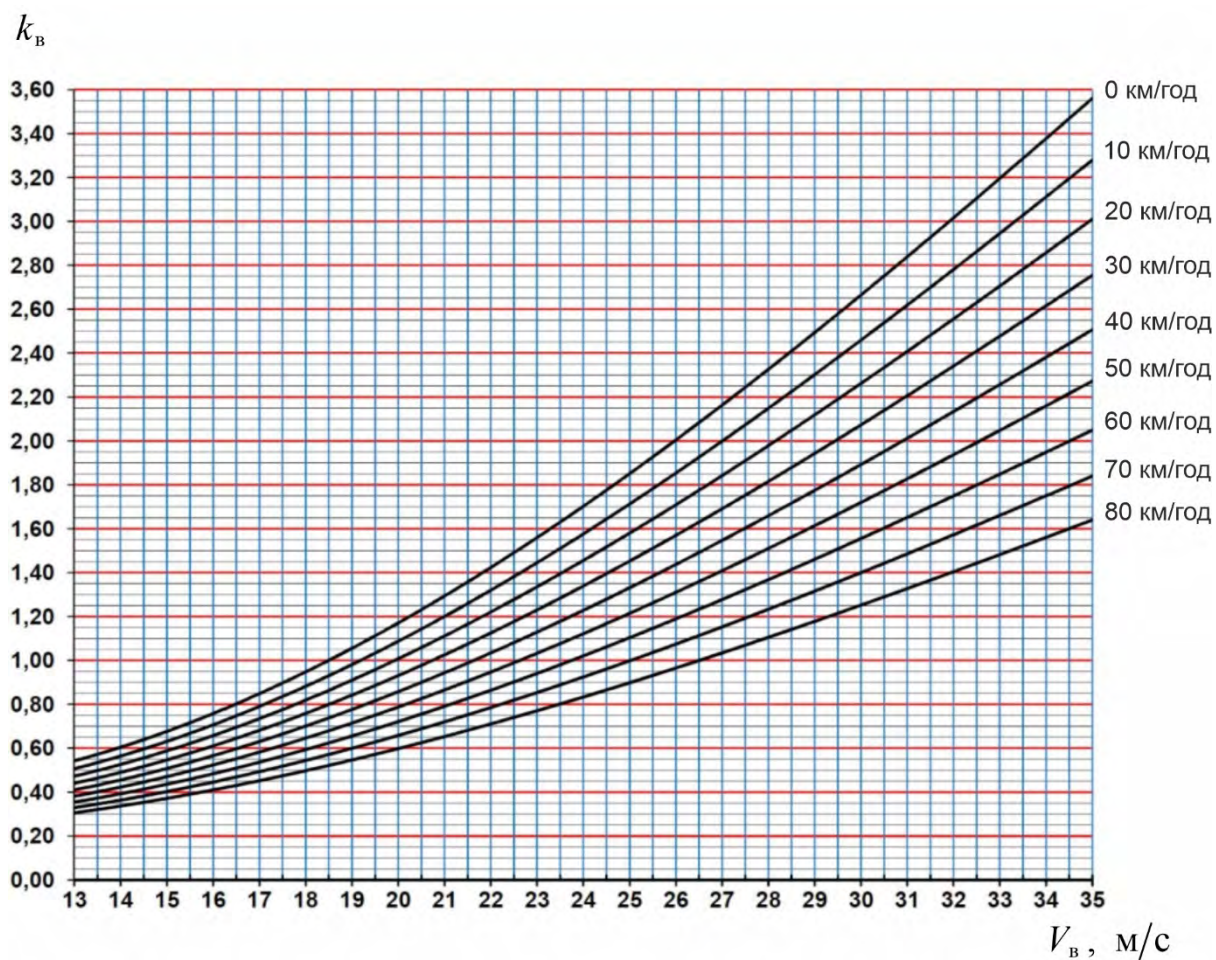
Рис. В.6. Номограма для визначення коефіцієнту k_B за швидкістю вітру від 13 до 35 м/с та густиною повітря 1,4 кг/м 3
