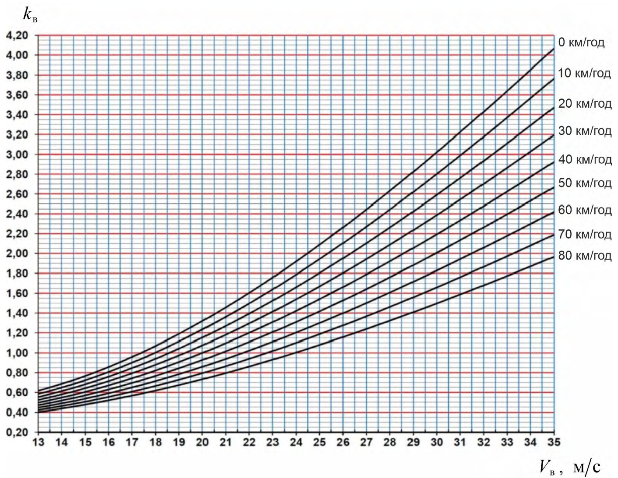
Рис. В.8. Номограма для визначення коефіцієнту k_B за швидкістю вітру від 13 до 35 м/с та густиною повітря 1,6 кг/м 3
