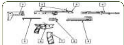
Іл. 19.16. Основні модулі карабіна А2
