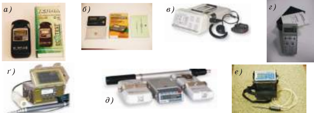
Іл. 42.8. Прилади для оснащення поста РХС:
