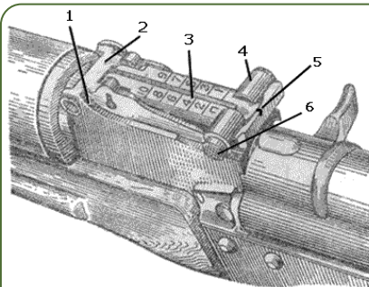
Іл. 20.4. Установка прицілу.
