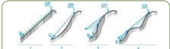
Іл. 30.10. Наявність взаємної видимості точок на одному схилі залежно від форми схилу
