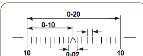
Іл. 29.3 б. Шкала бокових поправок оптичного прицілу ПСО-1
