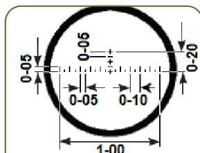
Іл. 29.3 а. Шкала бінокля, перископа
