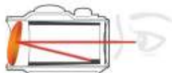
Іл. 20.15. Принцип дії коліматорних прицілів
