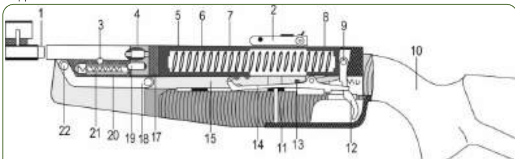
Іл. 24.4. Складові частини і механізми рушниці ІЖ-38: 1 — ствол; 2 — приціл; 3 — вісь ствола; 4 — прокладка ствола; 5 — коробка ствола; 6 — поршень; 7 — пружина бойова; 8 — колодка механізму спускового; 9 — штифт колодки; 10 — ложа; 11 — гвинт ложі задній; 12 — гачок спусковий; 13 — шептало; 14 — важіль блокування; 15 — важіль зведення; 17 — манжета; 18 — шарнір; 19 — клин; 20 — ригель; 21 — пружина ригеля; 22 — вісь шарніра
