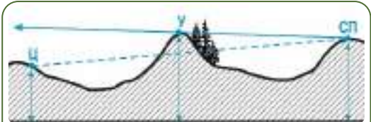
Іл. 30.8. Укриття вище спостерігача (СП) і цілі (Ц)
