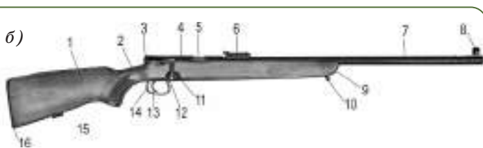
Іл. 24.1. Малокаліберна гвинтівка ТОЗ-8М, калібру 5,6 мм, з відкритим секторним прицілом: а) загальний вигляд; б) будова гвинтівки:
