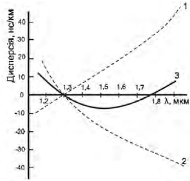
Рисунок 4.33 – Залежність дисперсійних характеристик ВОЛЗ від довжини хвилі
