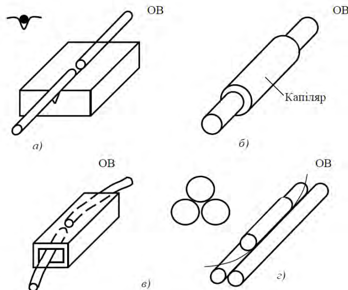
Рисунок 4.19 – Варіанти механічного з'єднання ОВ: а) У-подібна канавка; б) прецизійний капіляр; в) вільна трубка; г) три стрижні
