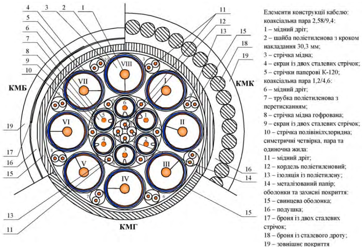
Рисунок 2.13 – Поперечний переріз кабелю КМ-8/6
