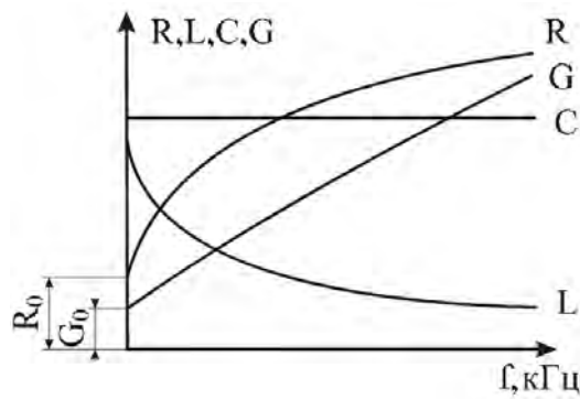
Рисунок 2.1 – Частотні характеристики первинних електричних параметрів симетричних ліній зв'язку
