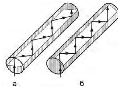
Рисунок 4.7 – Траєкторії поширення оптичних сигналів в ОВ
