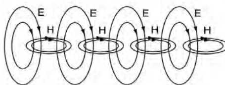
Рисунок 1.9 – Силкові лінії електромагнітного поля, що характеризують поширення енергії в напрямних системах електричного та оптичного зв'язку
