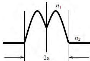
Рисунок 4.16 – Квазіпараболічний ППЗ багатомодових ОВ
