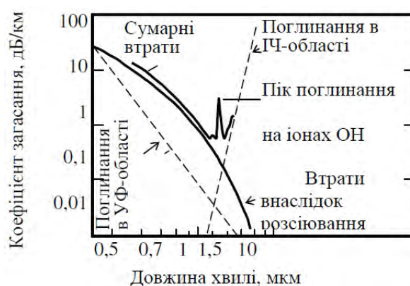
Рисунок 4.24 – Спектральна залежність коефіцієнта затухання кварцового ОВ, легованого германієм
