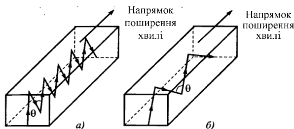
Рисунок 1.20 – Особливості поширення електромагнітної хвилі в хвелеводній напрямній системі
