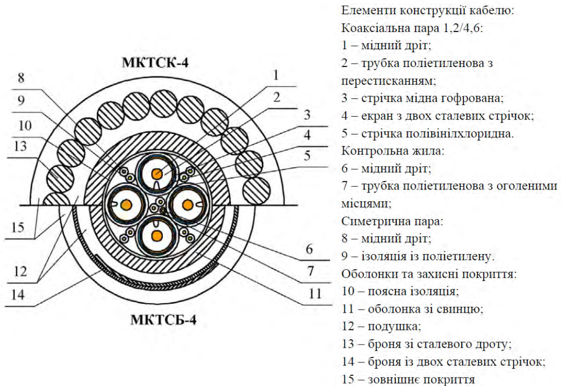
Рисунок 2.14 – Поперечний переріз кабелю МКТС
