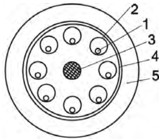
Рисунок 4.43 – Поперечний переріз ВОК міської ВОЛЗ
