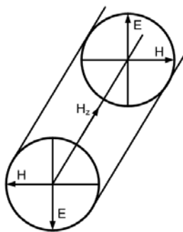
Рисунок 1.6 – Силкові лінії електромагнітного поля для ТЕ хвиль
