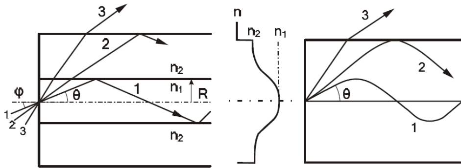
Рисунок 4.10 – Особливості поширення оптичних сигналів у ступінчастих та градієнтних хвильоводах
