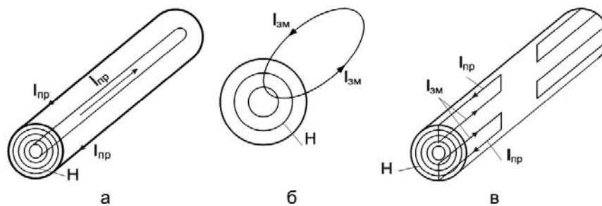
Рисунок 1.10 – Силові лінії струмів провідності та зміщення, що характеризують поширення енергії в напрямних системах електричного та оптичного зв'язку
