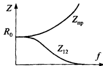
Рисунок 3.12 – Залежність опору зв'язку Z_{12} повного опору Z_{np} зовнішнього провідника коаксіального кабелю робочої частоти
