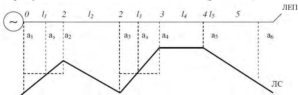
Рисунок 3.14 – Траса зближення
