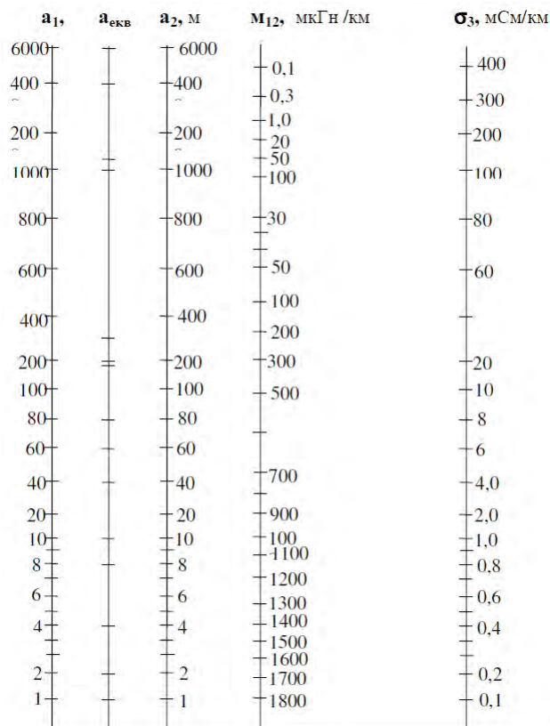
Рисунок 3.15 – Номограма Михайлова
