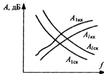
Рисунок 3.13 – Залежності перехідних затухань між коаксіальними та симетричними колами на ближньому та дальньому кінцях лінії електрозв'язку
