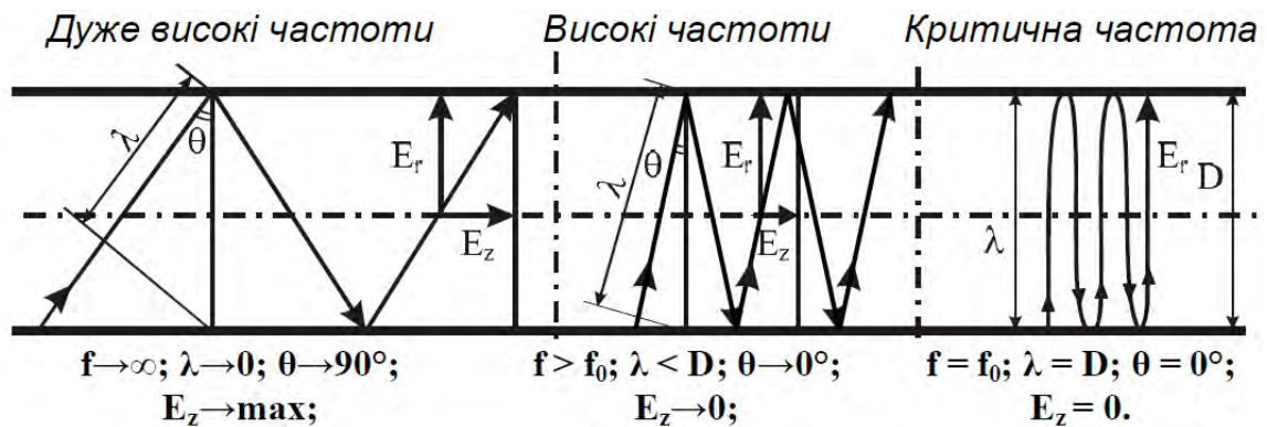
Рисунок 4.3 – Класифікація режимів поширення хвиль оптичним хвильоводом
