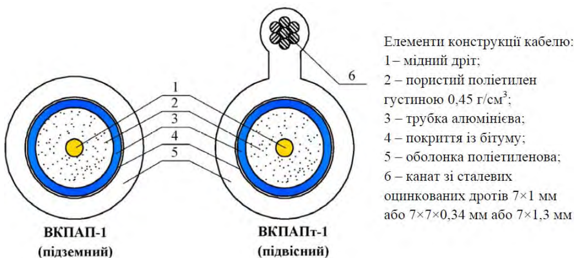
Рисунок 2.15 – Поперечний переріз кабелю ВКПАП-1 та елементи його конструкції
