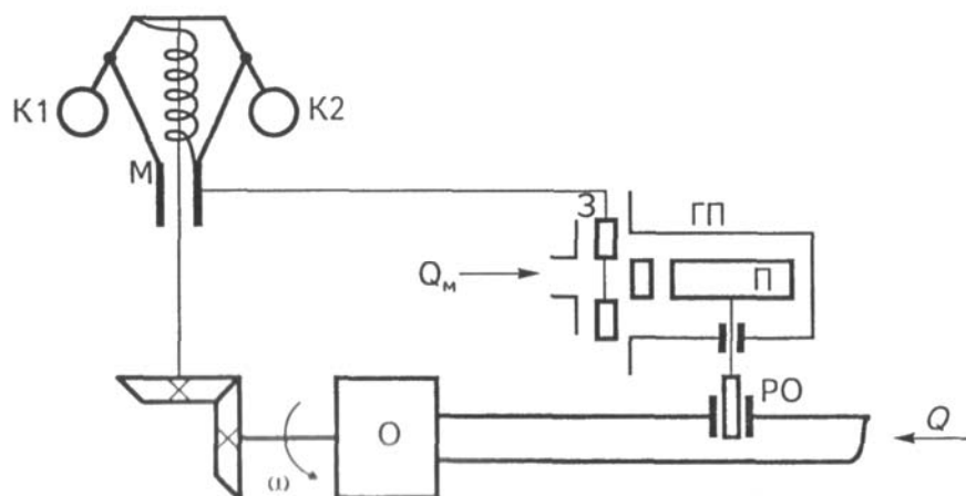
Рис.1.6. САР непрямої дії регулювання швидкості об'єкта
