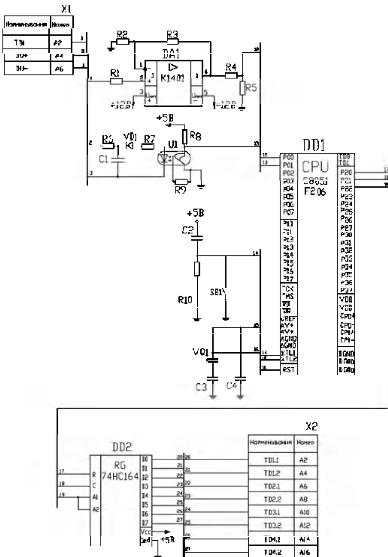
Рис. 11.13. Принципова електрична схема
