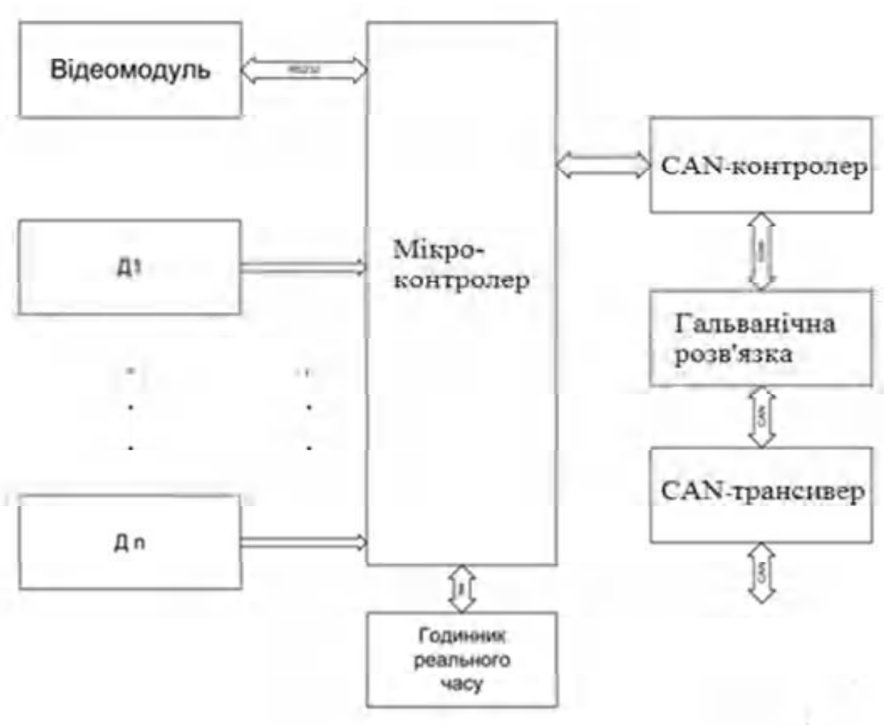
Рис. 11.8. Структурна електрична схема
