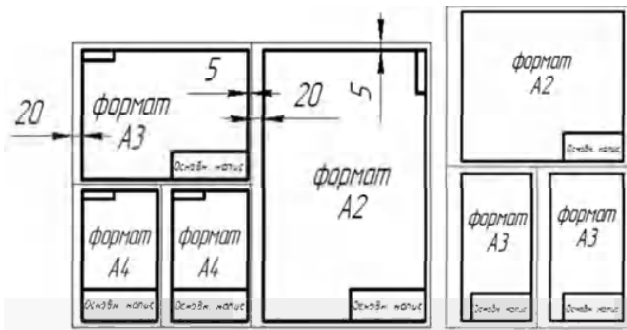
Рис. 11.2. Розташування декількох креслень на аркуші формату A1
