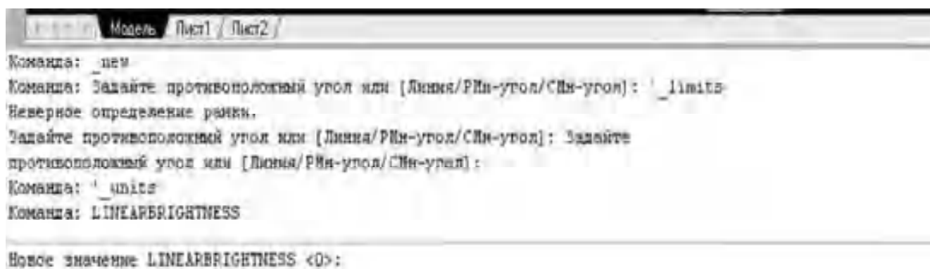
Рис. 5.2. Вікно команд
