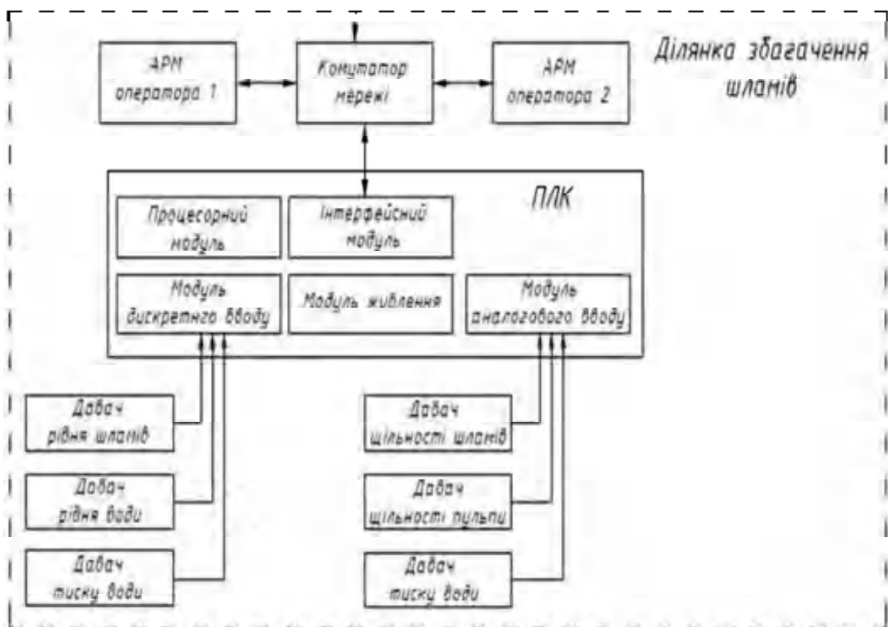
Рис. 11.9. Структурна схема комплексу технічних засобів комп'ютерної системи
