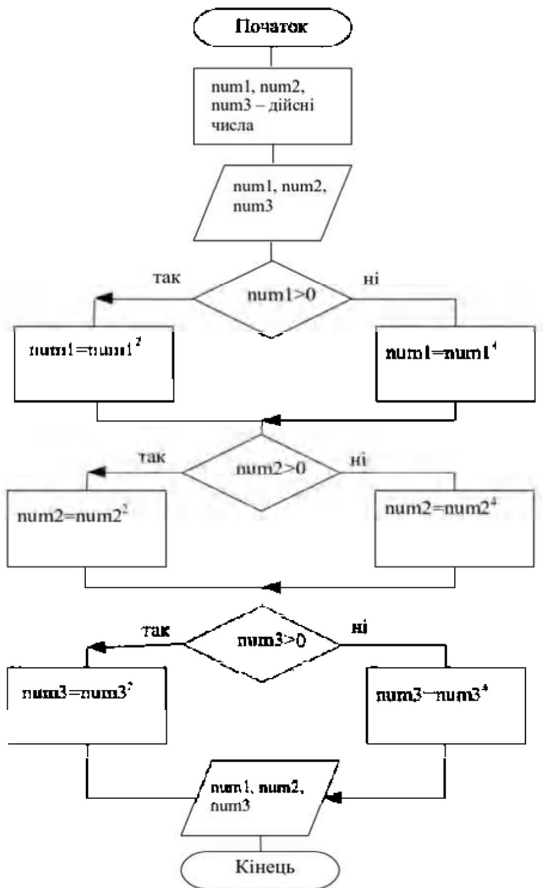
Рис. 10.2. Схема програми прикладу
