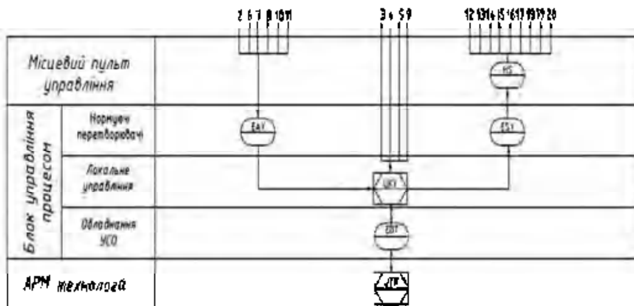
Рис. 11.11. Функціональна схема автоматизації
