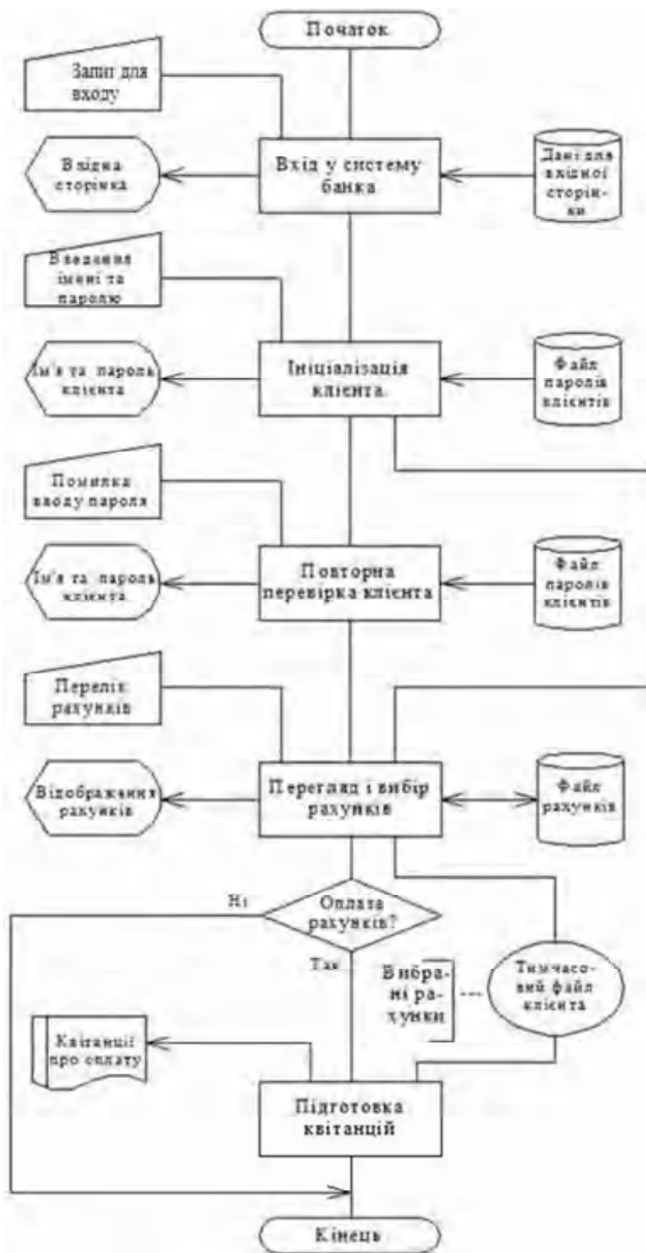
Рис. 10.3. Схема алгоритму роботи комп'ютерної системи
